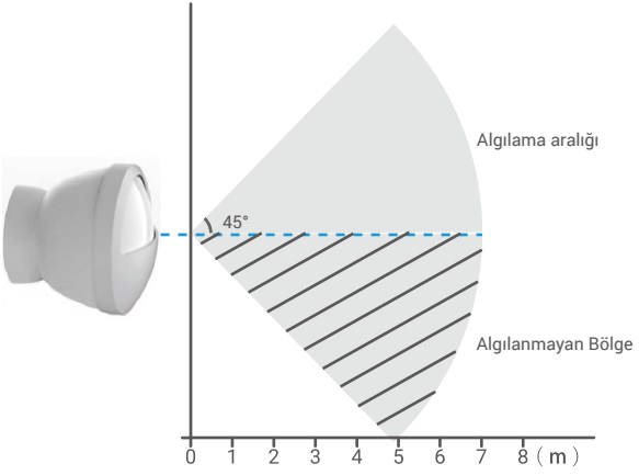
Şekil 2 Algılama aralığının üstten görünümü
